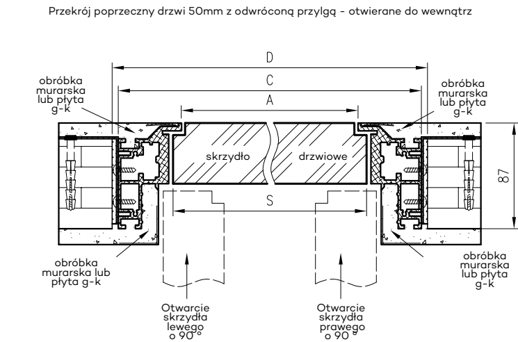
Wymiary szerokości drzwi Profi
