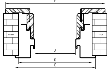
Profil ościeżnicy
