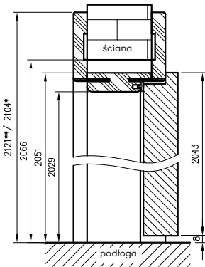
Przekrój pionowy drzwi przylgowych z OR
