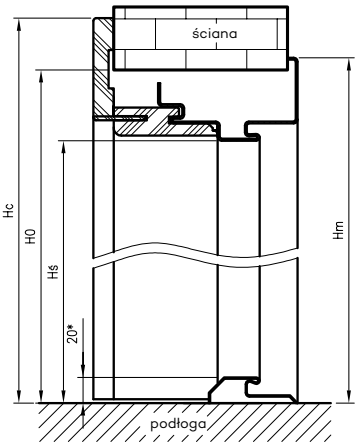
Wymiary OSH STAND dla drzwi dwuskrzydłowych
