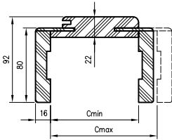
Przekrój OR z ką. T80
