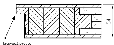
Skrzydło drzwiowe antywłamaniowe - przeciwpożarowe NEFRYT RC2/RC3 EI-30
