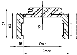
Przekrój OR/ORC z kąt. T63
