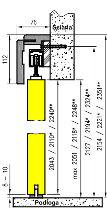
NS - przekrój pionowy
