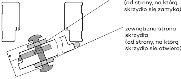
Rys. Dobór wymiaru wkładki z gałką
