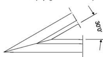
Minimalny kąt dla ramy i skrzydła
