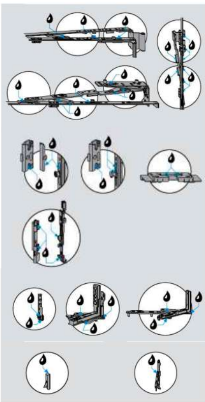
Miejsca smarowania okuć Siegenia
